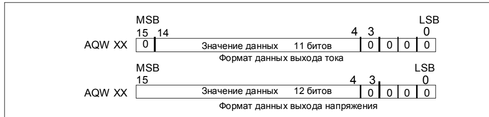
Рис. А-23. Формат выходного слова данных для 232 и EM 235
