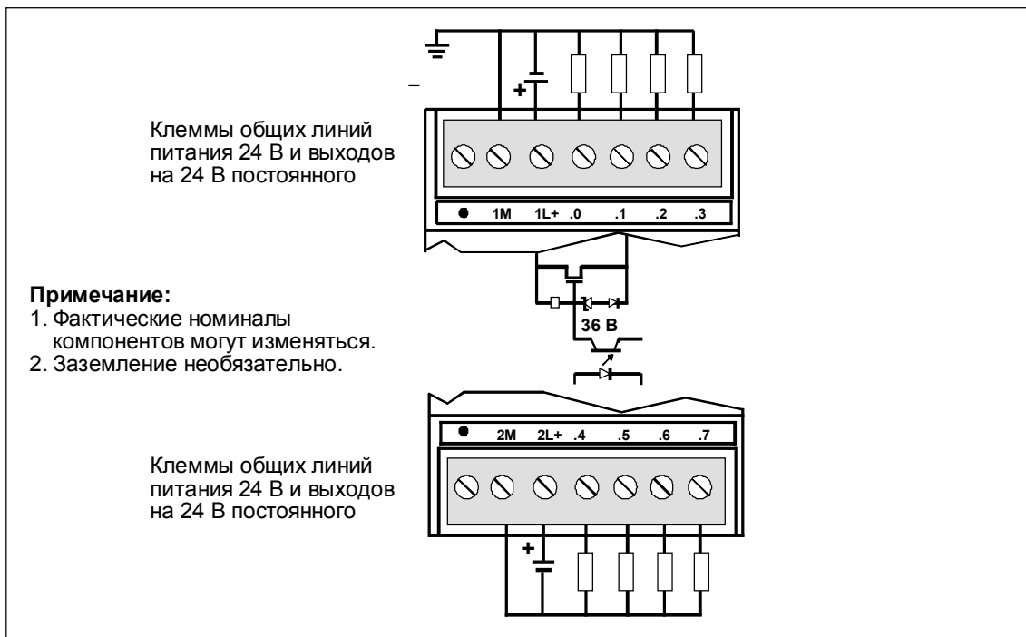
Рис. А-11. Обозначение клемм соединительной колодки для EM 222 Digital Output 8 x 24 VDC
