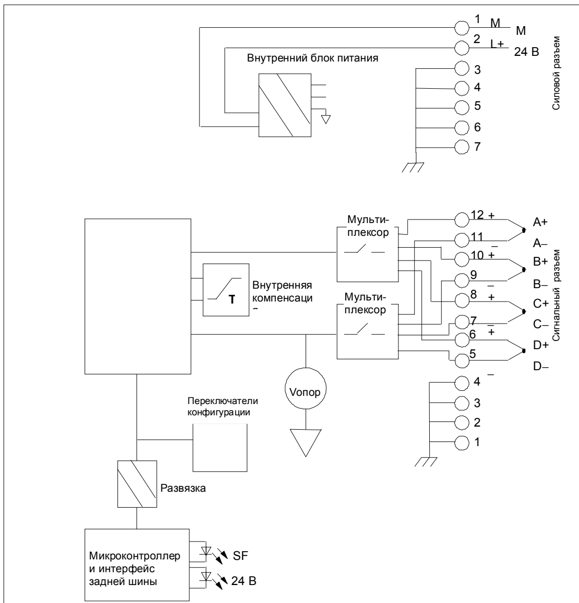
Рис. А–36. Принципиальная электрическая схема модуля с термопарой
