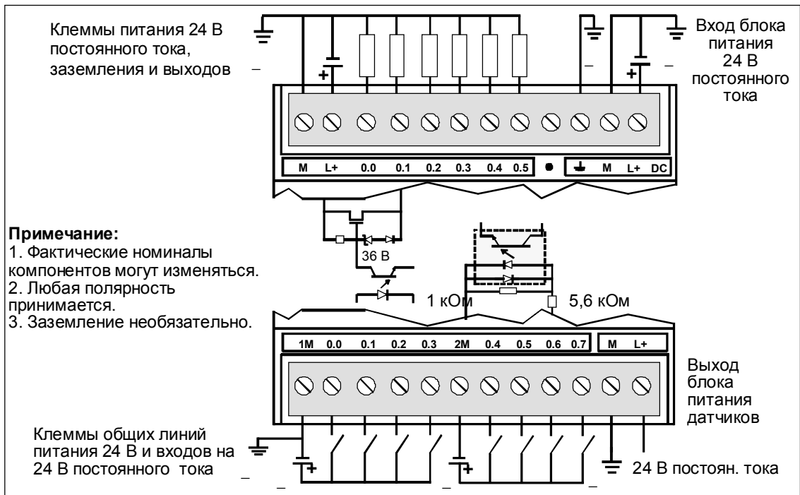
Рис. А-4 Обозначение клемм соединительной колодки для CPU 222 DC/DC/DC
