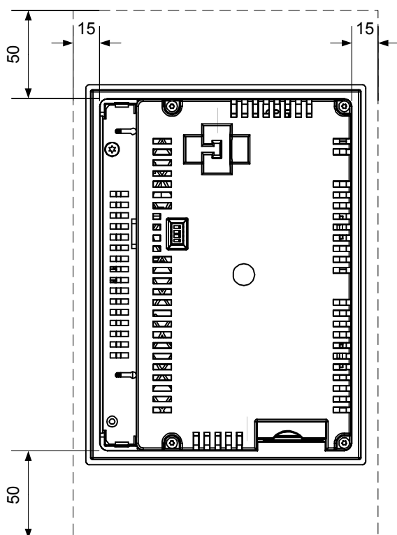
Рисунок 3-8 Зазоры при установке устройства НМИ
