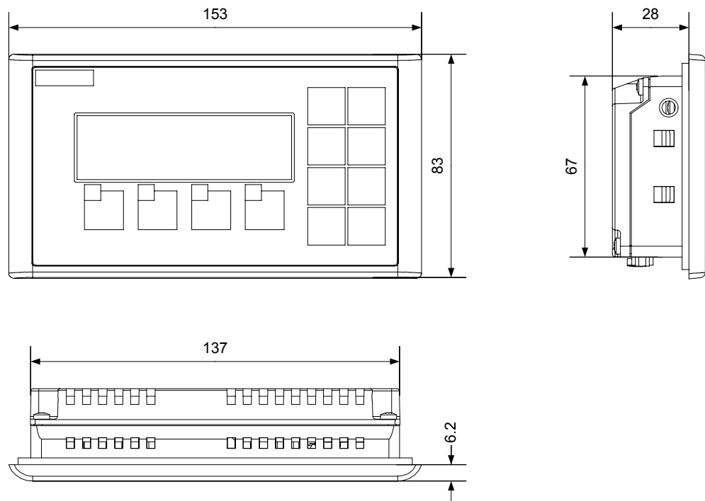
Рисунок 11-1 Габаритные размеры устройства HMI
